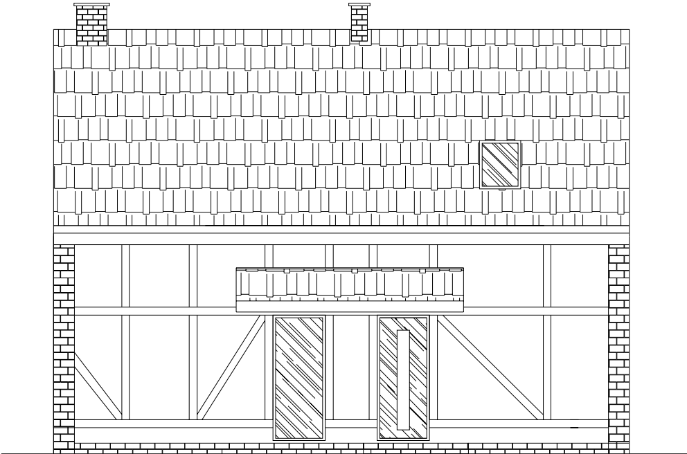
ELEWACJA POŁUDNIOWO-ZACHODNIA
