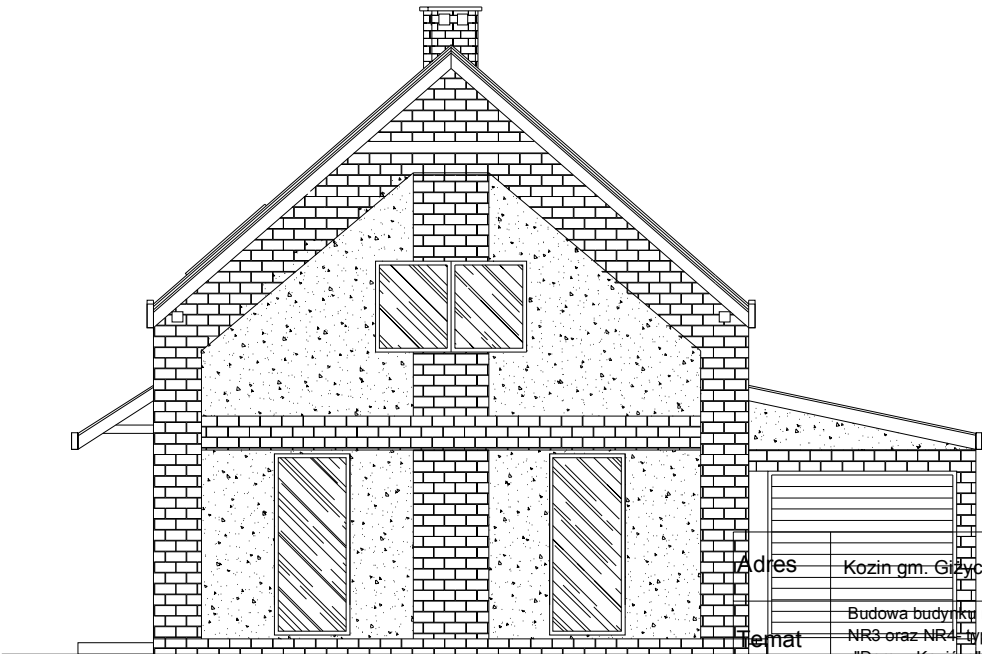
ELEWACJA POŁUDNIOWO-WSCHODNIA
